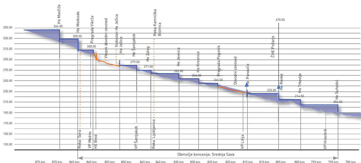
Hidroelektrarne na srednji Savi Podolžni profil - informativni prikaz
